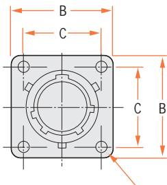
4 trous/holes Ø 3,15 +0,15 tailles/sizes 8 à/to 22
